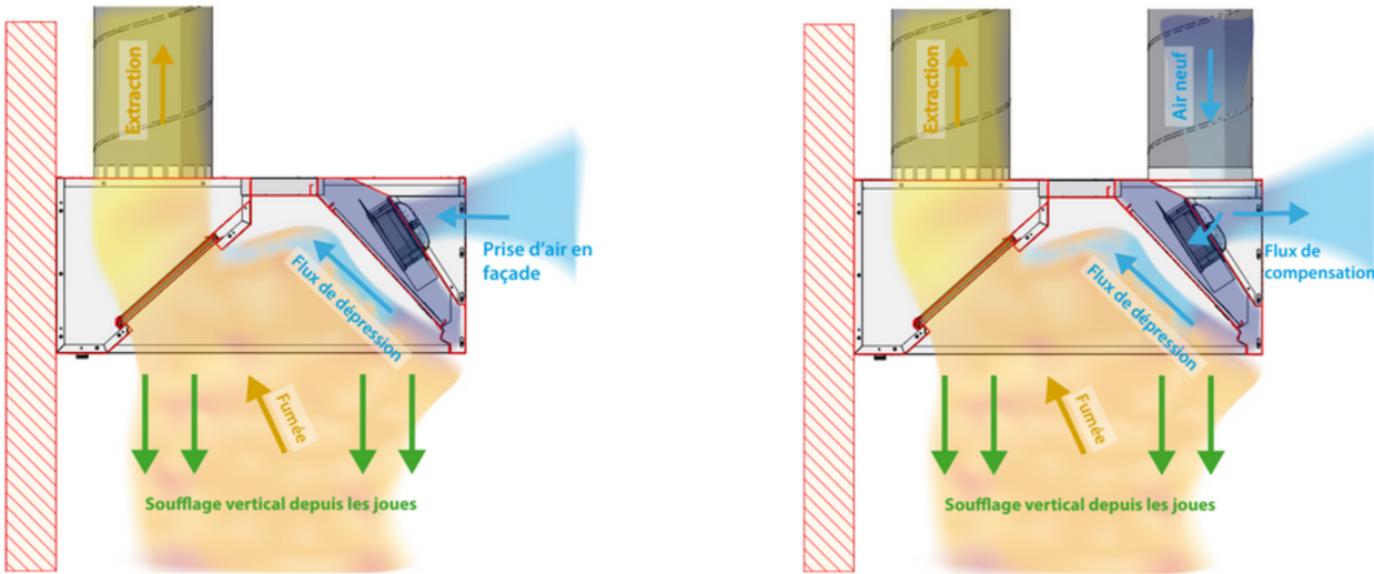
Principe du système IDFi avec soufflage joue
